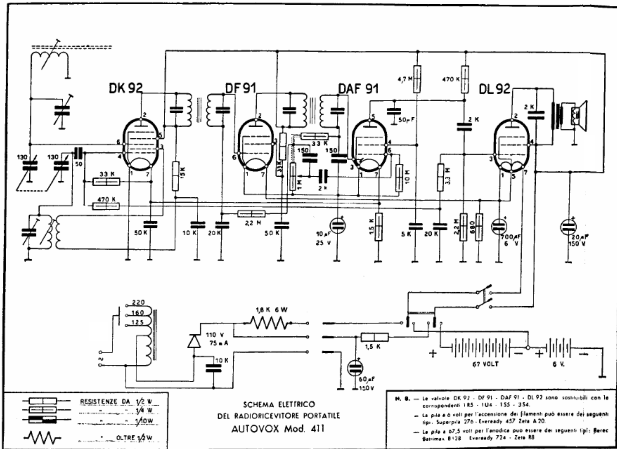
AUTOVOX - Mod. 411. Portatile alimentabile a pile e a corrente alternata. Gamma onde medie da 540 a 1600 kc/s. Dimensioni: 21×15×6 cm. Peso 1900 grammi. MF a 455 kc/s.
